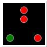
תמונה 66 כלי שיט ללא שליטה, עושה דרכו במים, מבט מלפנים
