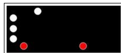
תמונה 59 כלי שיט גורר ונגרר עם משך שאורכו קטן מ- 200 מטר מוגבל בכושרו לתמרן, מפליגים ימינה
