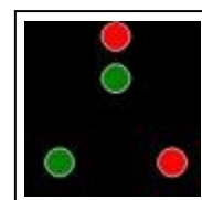
תמונה 58 מפרשית שאורכה מעל 20 מטר (עושה דרכה במים), מבט מלפנים
